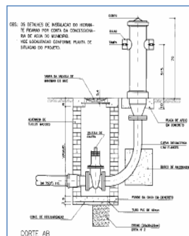
Esquema de Hidrante de Coluna Urbano
